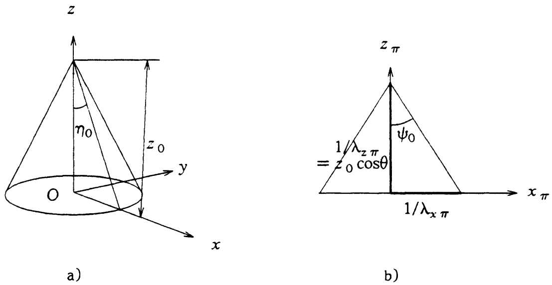
Fig.4.4. a) Circular Cone. b) Silhouette.
